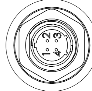
DETAIL Y 2 : 1
